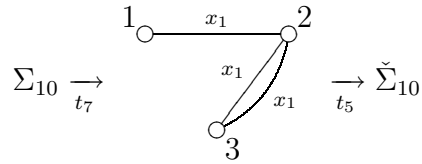
Рис. 8.6: вывод t_{10}
