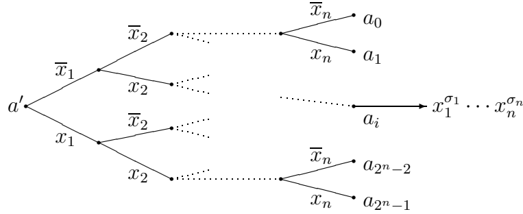
Рис. 5.4: контактное дерево
