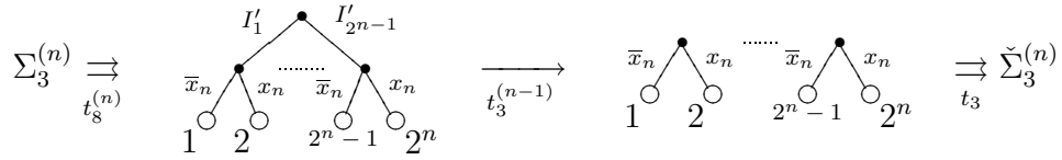
Рис. 8.10: вывод t_3^{(n)}
