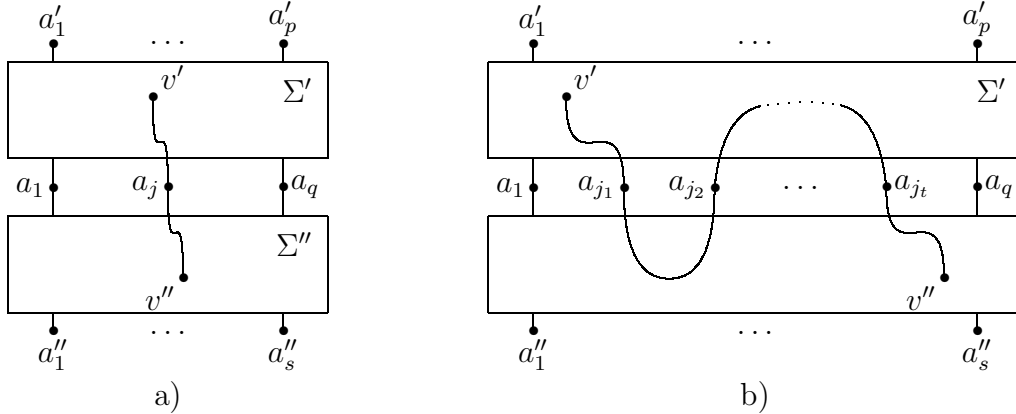
Рис. 6.2: к доказательству леммы 6.1
