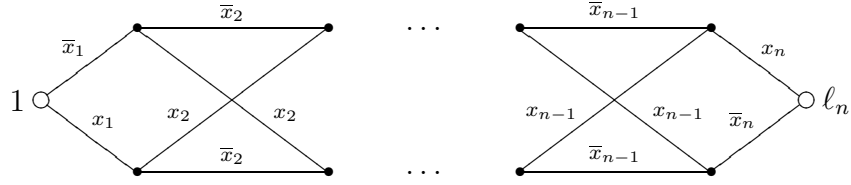
Рис. 2.6: схема Карно для линейной функции \ell_n
