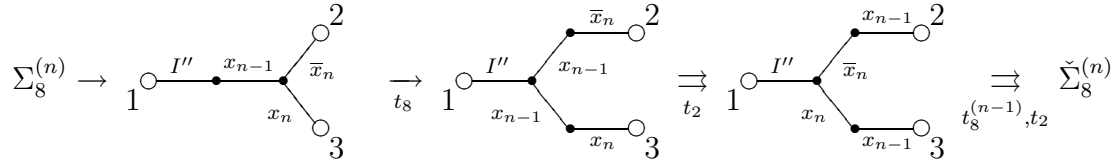
Рис. 8.9: вывод t_8^{(n)}
