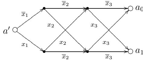
Рис. 7.7: BDD для \ell_3
