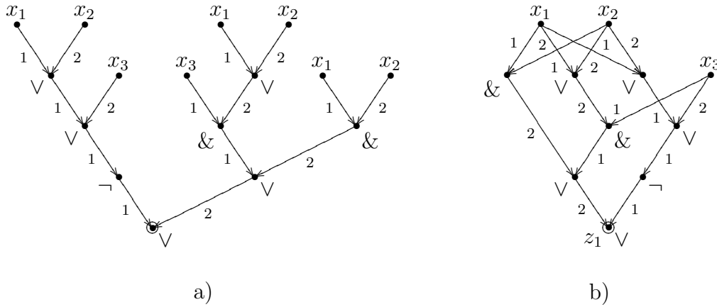
Рис. 2.3: представление формулы (2.3) деревом и квазидеревом
