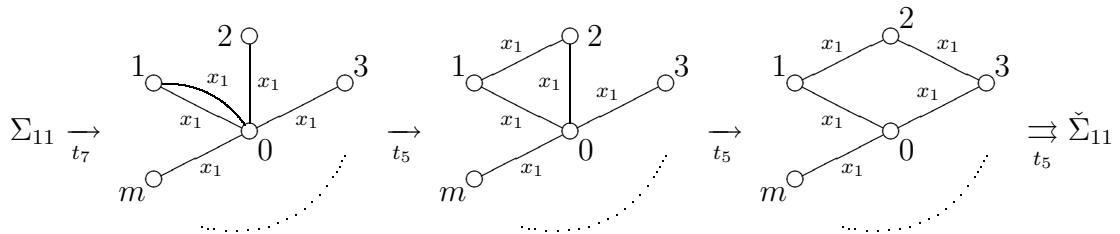
Рис. 8.7: вывод t_{11}
