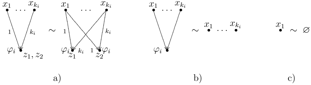
Рис. 10.2: тождества ветвления, снятия \Phi\Delta и снятия входа
