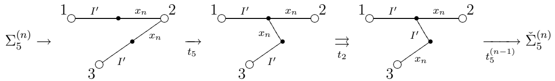
Рис. 8.12: вывод t_5^{(n)}
