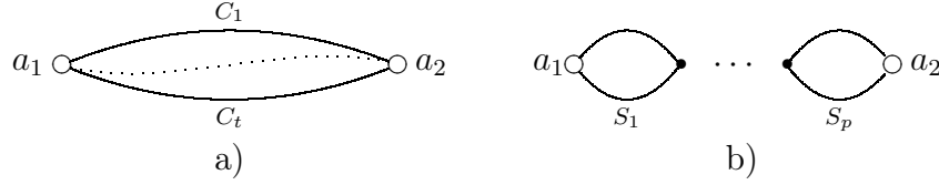
Рис. 5.5: КС, моделирующая ДНФ и КНФ
